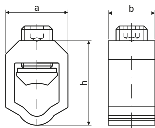
25-120SW
