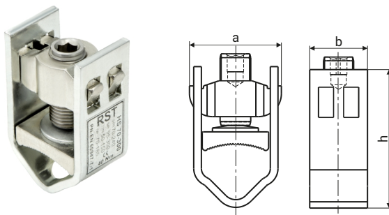
HS 70-300
