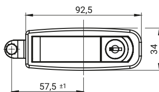
2.615.004
