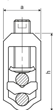
2/25-120SW-B 2/25-120SW-E
