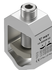
10-300SW-02
