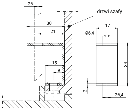
ROD GUIDE Ø6 - U 1C.906.001
