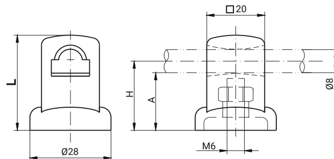
ROD GUIDE Ø8 1C.906.008, 1C.906.009, 1C.906.010
