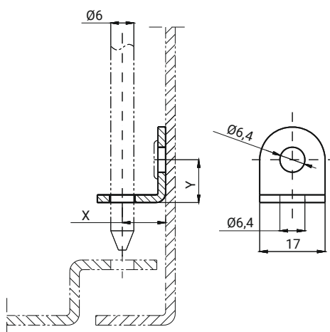
ROD GUIDE Ø6 - L 1C.906.002
