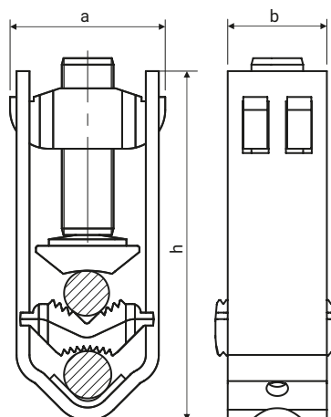
HS 2/50-240-D
