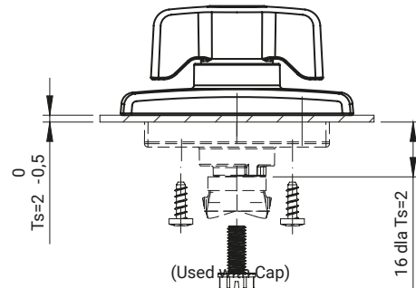
RW505.N
