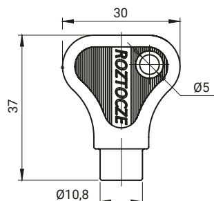
2.KLB-X.002
