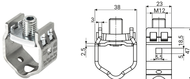
HS 120-300
