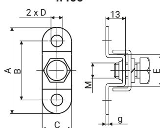
ЗАЖИМ 4-ВИНТОВЫЙ 4.406
