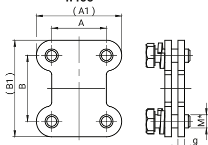
ЗАЖИМ 4-ВИНТОВЫЙ 4.405
