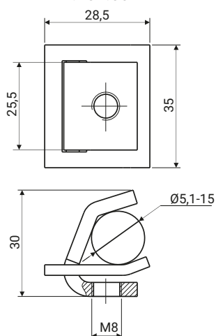
ЗАЖИМ ЛИНЕЙНЫЙ ДЛЯ ГОЛОЙ ЛИНИИ 4.402.001
