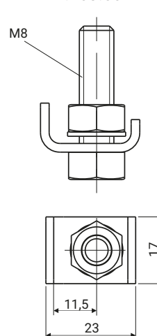
ЗАЖИМ ЗАЗЕМЛЯЮЩИЙ 4.403.001
