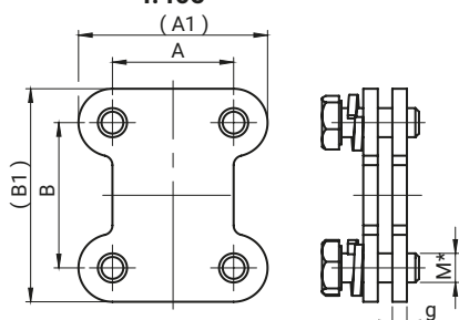
ZACISK 4-ŚRUBOWY 4.405
