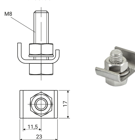
ZACISK UZIEMIĄJĄCY 4.403.001
