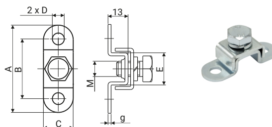
ZACISK UZIEMIĄJĄCY 4.406
