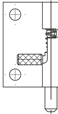
Петля правая 3.ST79.001
