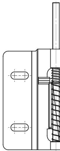
Петля правая 3.ST104.006.001
