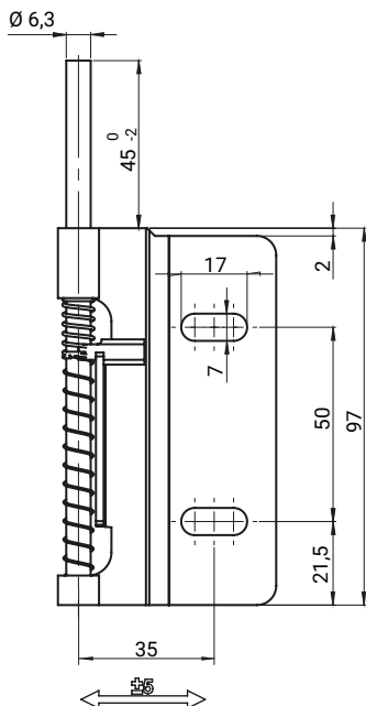
Петля левая 3.ST104.006.002
