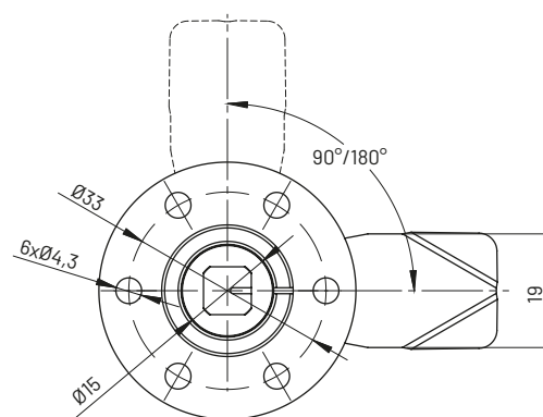
M22K / M22K15
