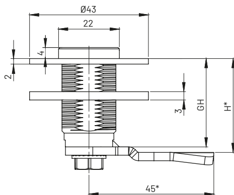
M22KW
