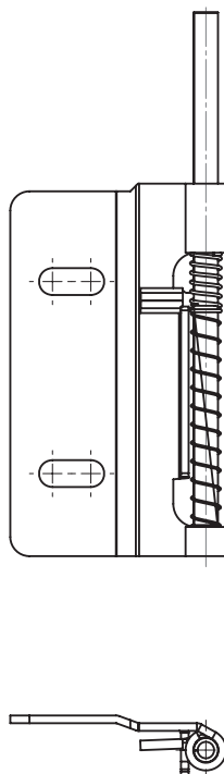
Петля правая 3.ST104.006.001
