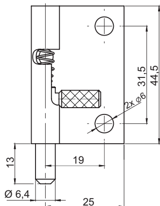
Петля левая 3.ST79.002
