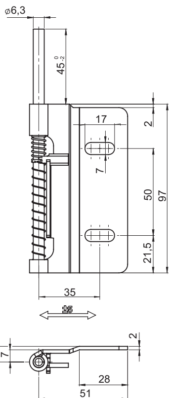
Петля левая 3.ST104.006.002
