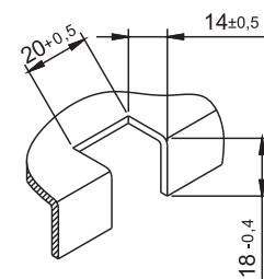
Otwór montażowy
