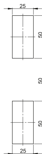
Otwór montażowy
