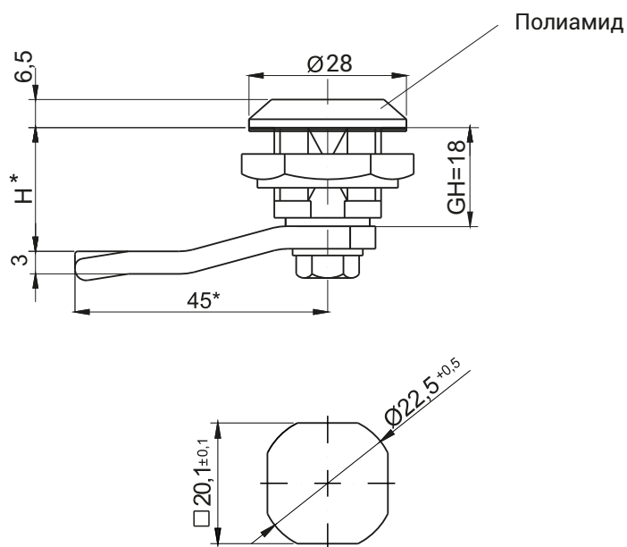
Монтажное отверстие
