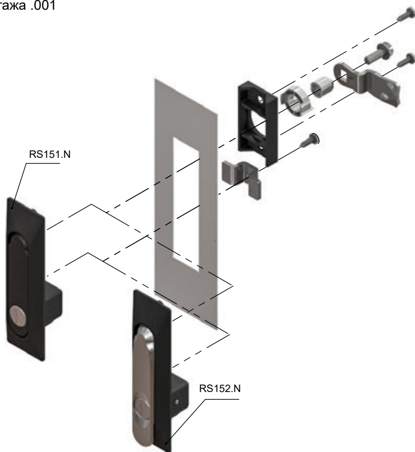
Способ монтажа .001
