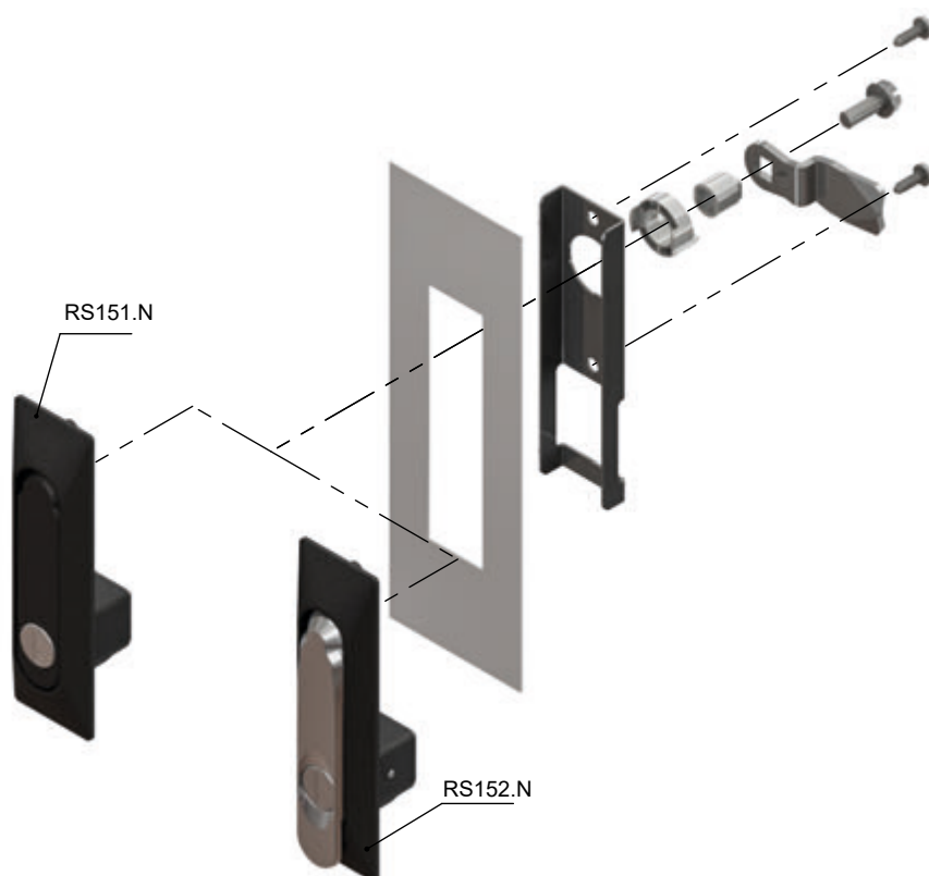
Способ монтажа .002
